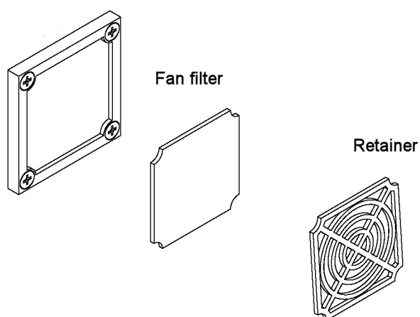
Fig. 83 Removing the fan filter
